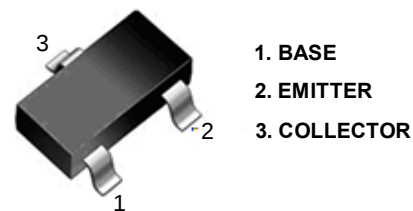
SOT - 23
