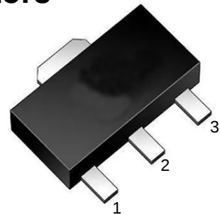
SOT-89-3L
