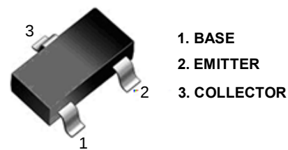
SOT - 23
