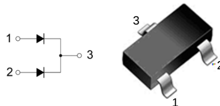
SOT - 23
