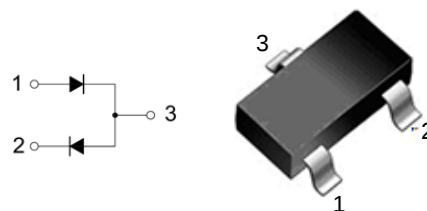
SOT - 23
