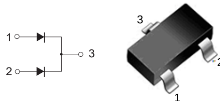
SOT - 23
