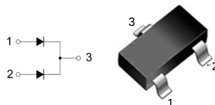
SOT - 23
