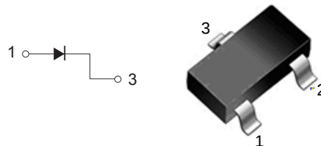
SOT - 23
