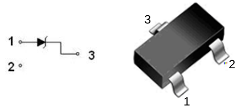
SOT - 23
