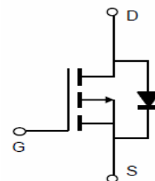
P-Channel MOSFET
